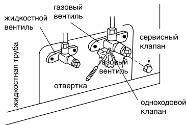
Рис. 9 жидкостной вентиль
